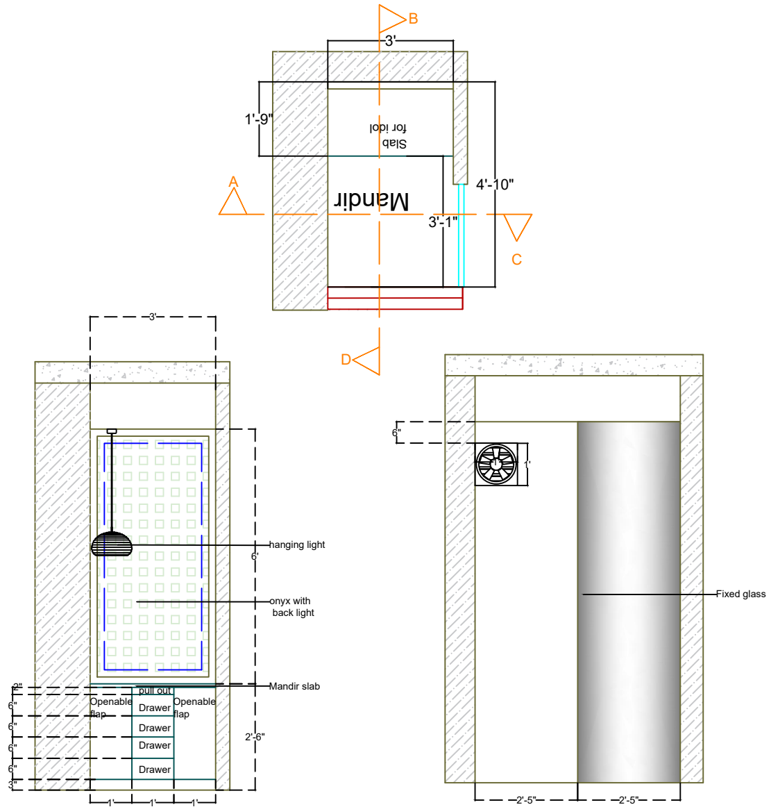
Elevation A
