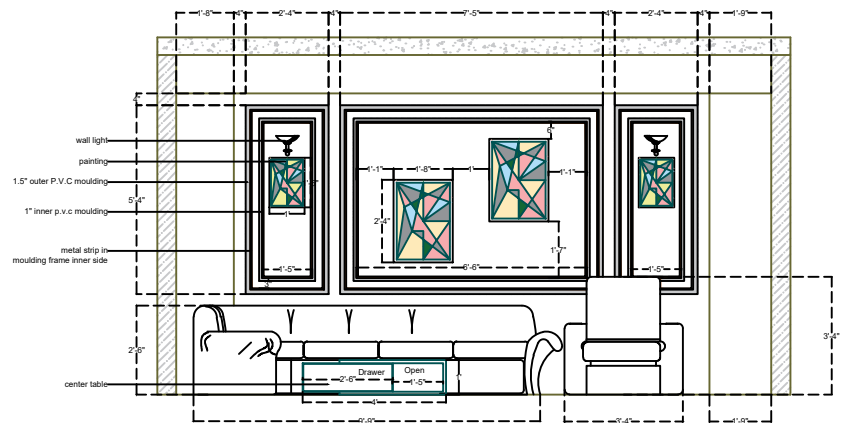
Elevation B
