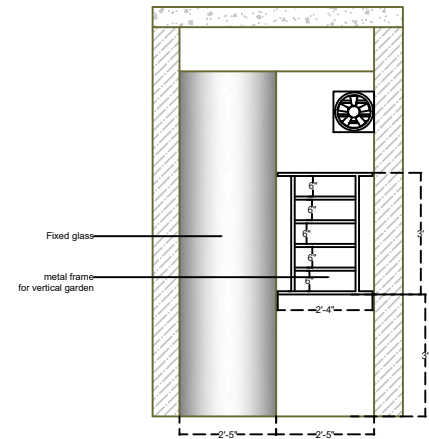
Elevation B
