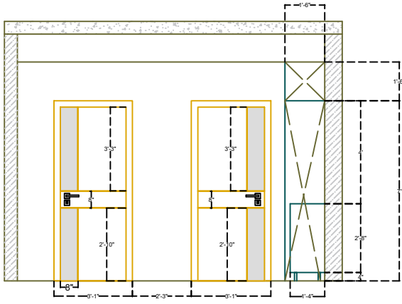
Elevation A
