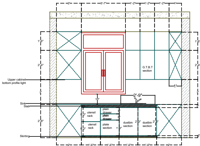
Elevation A
