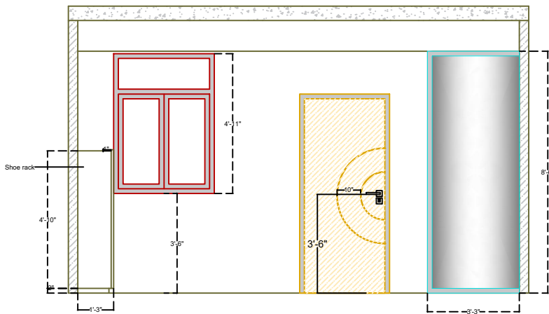
Elevation A
