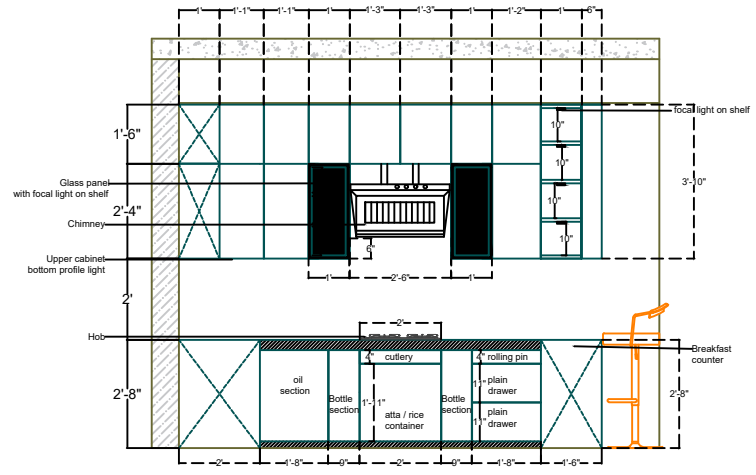
Elevation B
